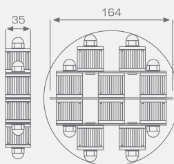
Tipo PMTO per tramogge coniche tonde Type PMTO for use with conical hopper Type PMTO für konische Trichter Type PMTO pour trémies coniques rondes
