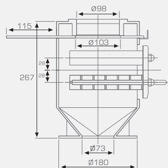
Tipo 110 con paratia mobile Type 110 with slide gate Type 110 mit Absperrschieber Modèle 110 avec trappe coulissante
