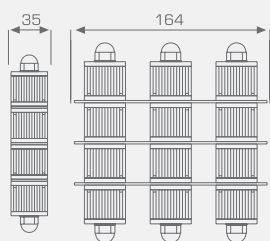
Tipo PMQO per tramogge quadre Type PMQO for use with square hopper Type PMQO für quadratische Trichter Type PMQO pour trémies carrées
